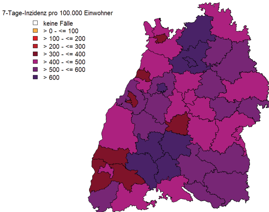
Abbildung 3: 7-Tage-Inzidenz der übermittelten COVID-19-Fälle pro 100.000 Einwohner nach Meldelandkreis, Baden-Württemberg, Stand: 08.12.2021, 16:00 Uhr.
